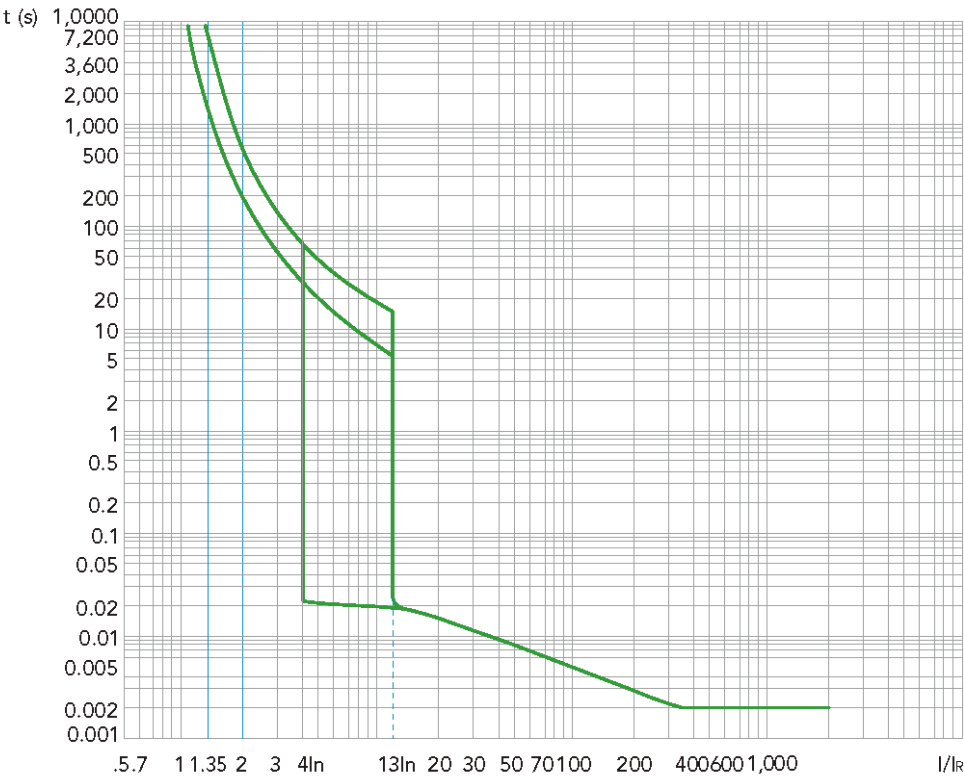
M3 (225~350 A)
