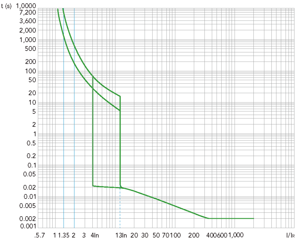
M3 (400 A)
