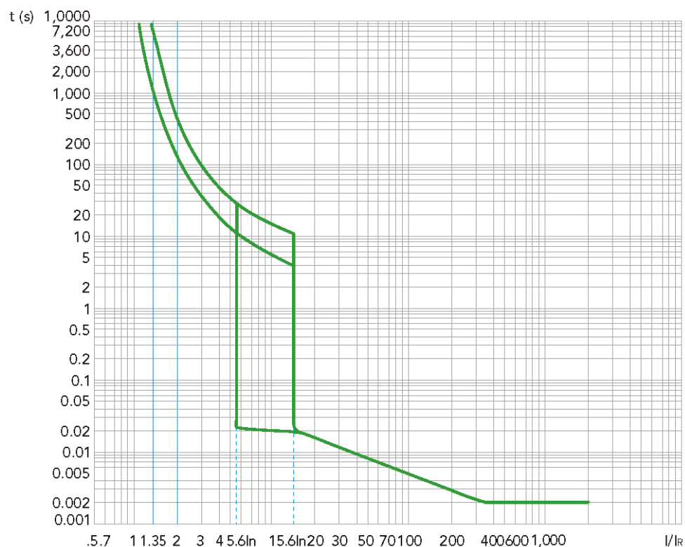
M2 (100~150 A)
