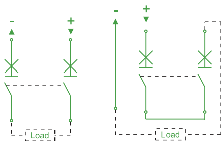
2 Poles
