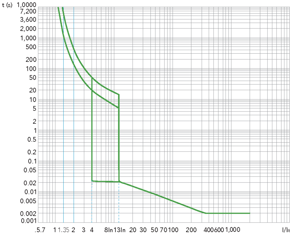
M1 (125~150 A)
